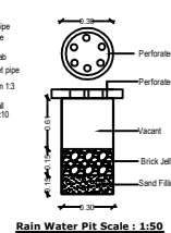
Rain Water Pit Scale: 1:50
