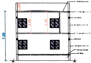
SECTION 'AB'
