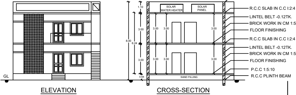
ELEVATION
