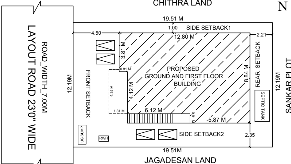
SITE PLAN-SCALE=1:100
