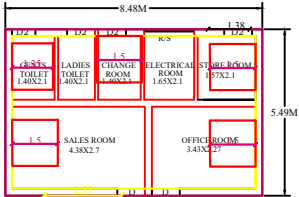
PLAN( NTS)
