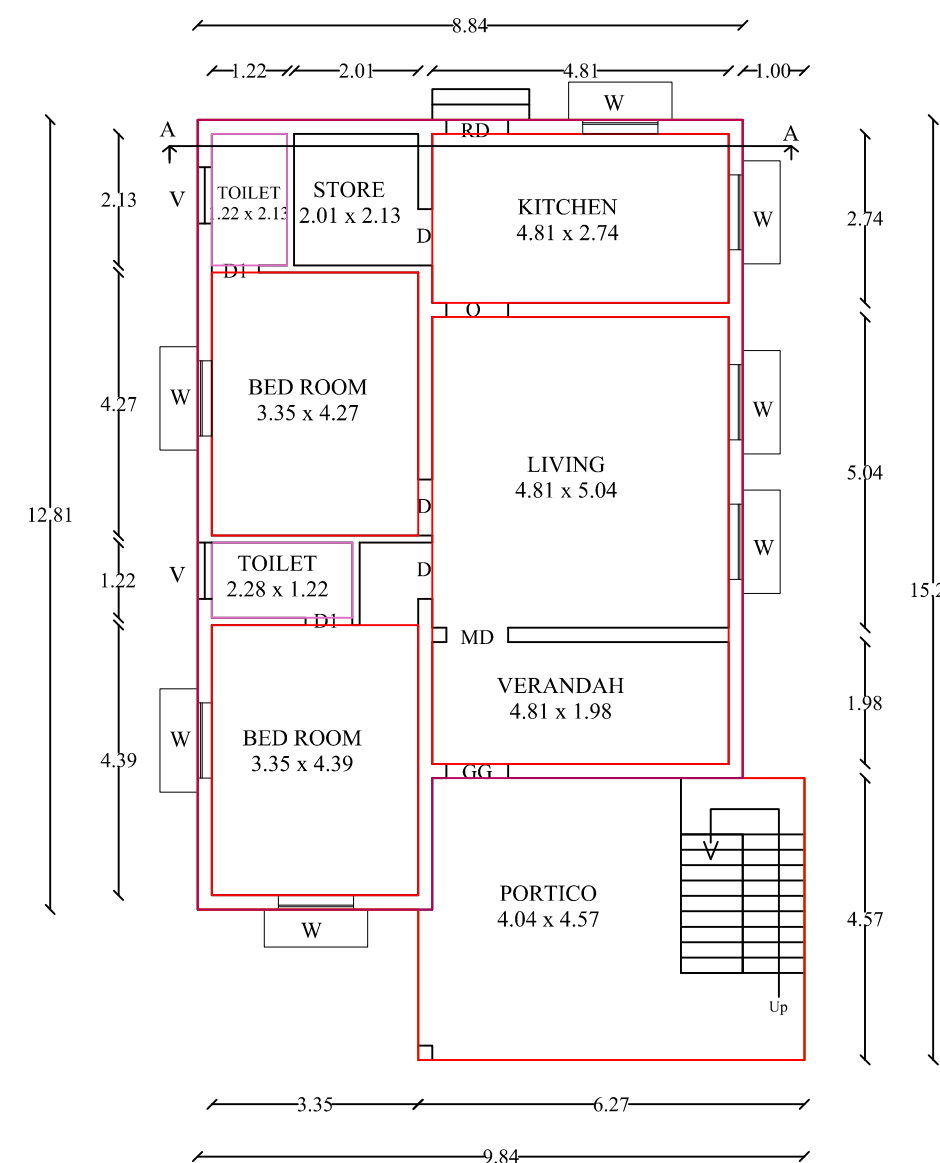
UND FLOOR PLAN
