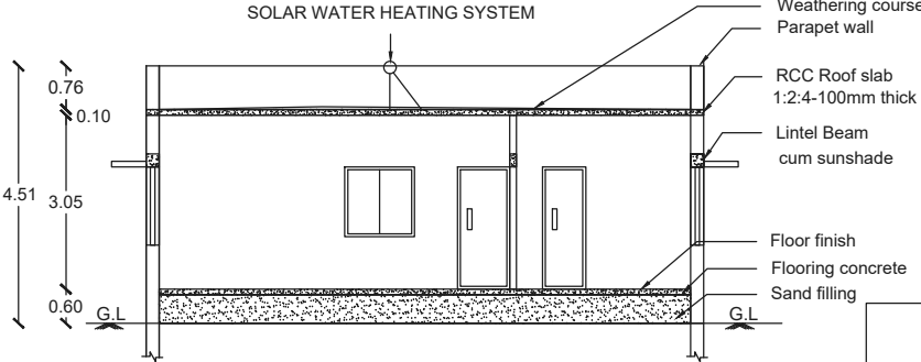
SECTION ON DE
