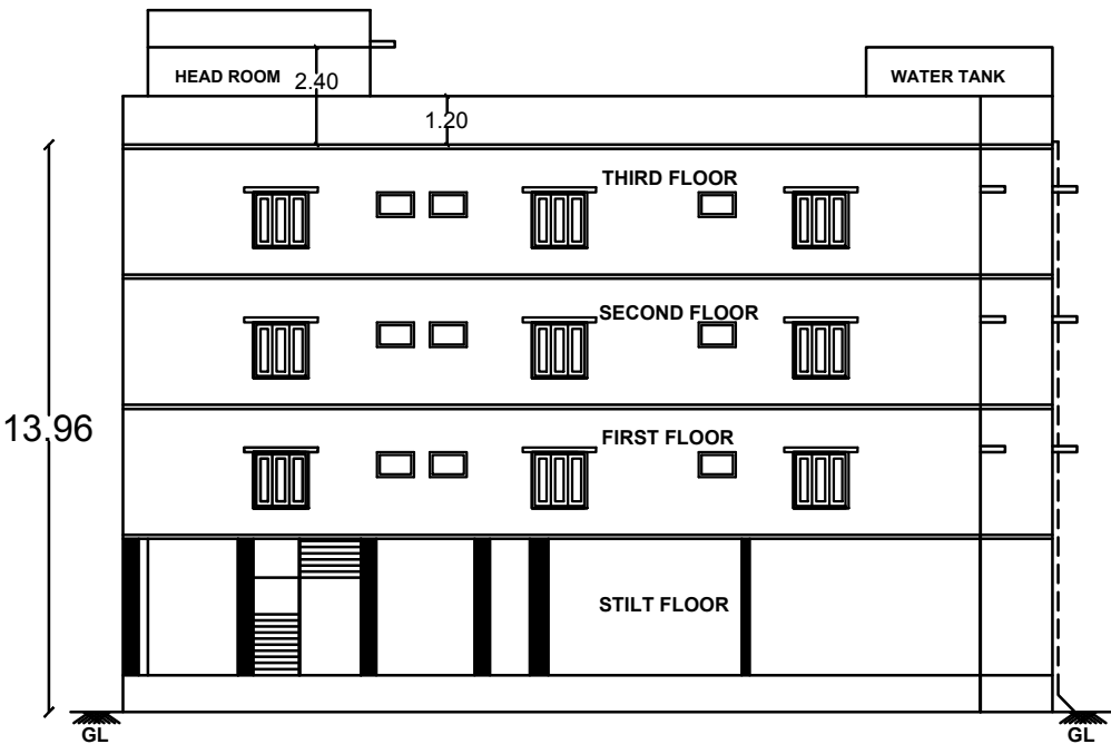
ELEVATION
