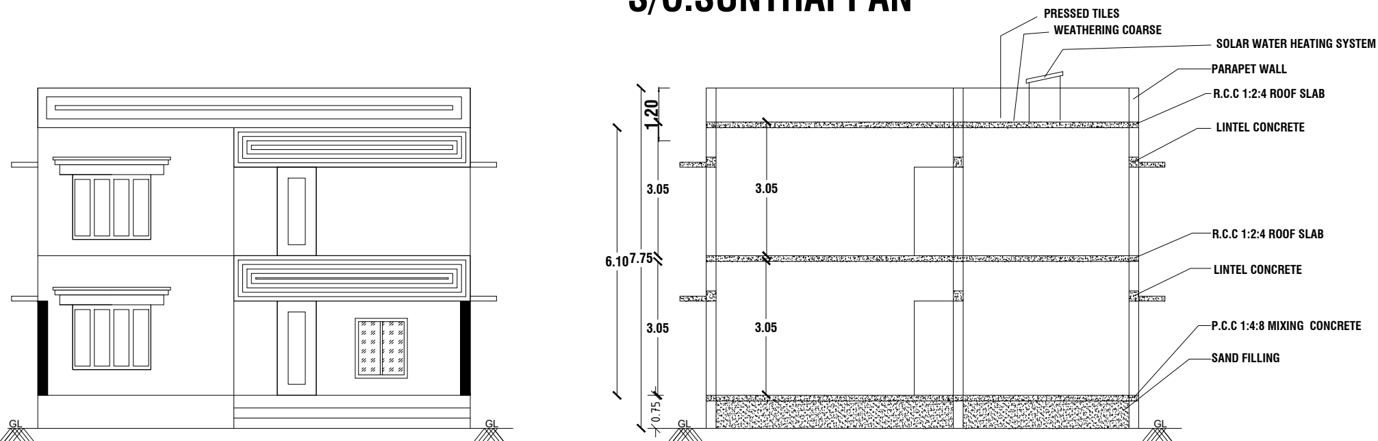
ELEVATION
