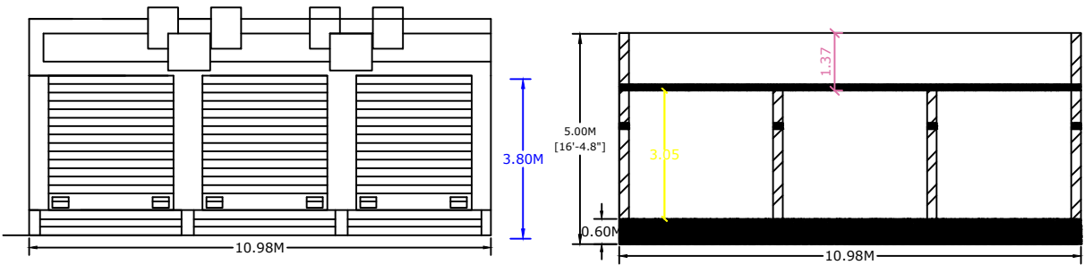
ELEVATION
