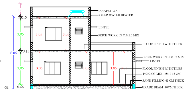
SECTION A-B
