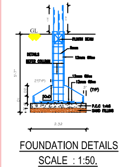
SCALE : 1:50.
