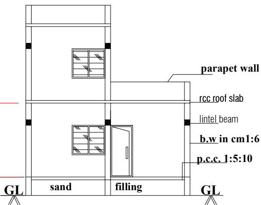
SECTION 'AB'
