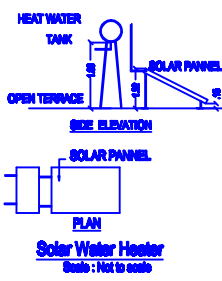
Solar Water Heater Scale: 1:50
