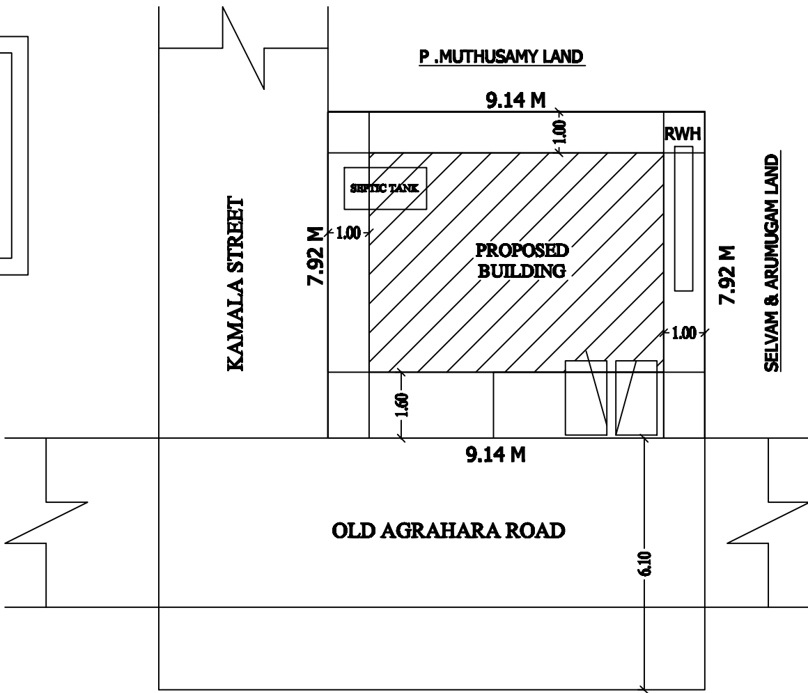
SITE PLAN 1:100
