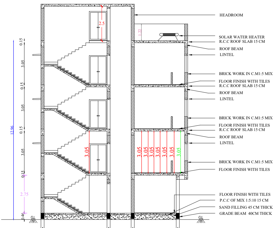
SECTION:A-B
