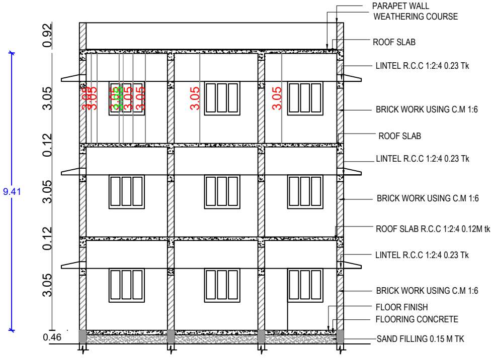
SECTION A-C
