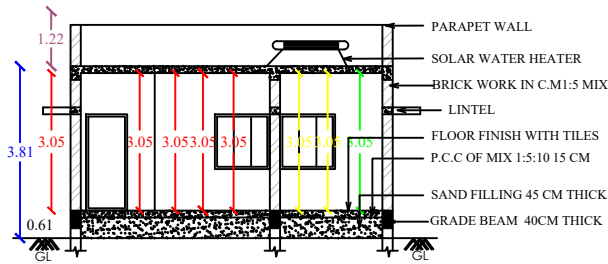
SECTION A-B
