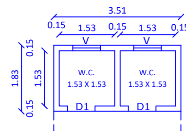
TOILET PLAN
