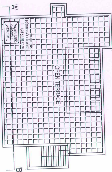
PRO. TERRACE PLAN.
