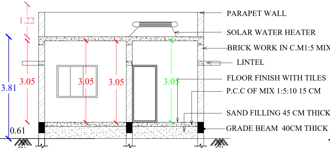
SECTION A-B
