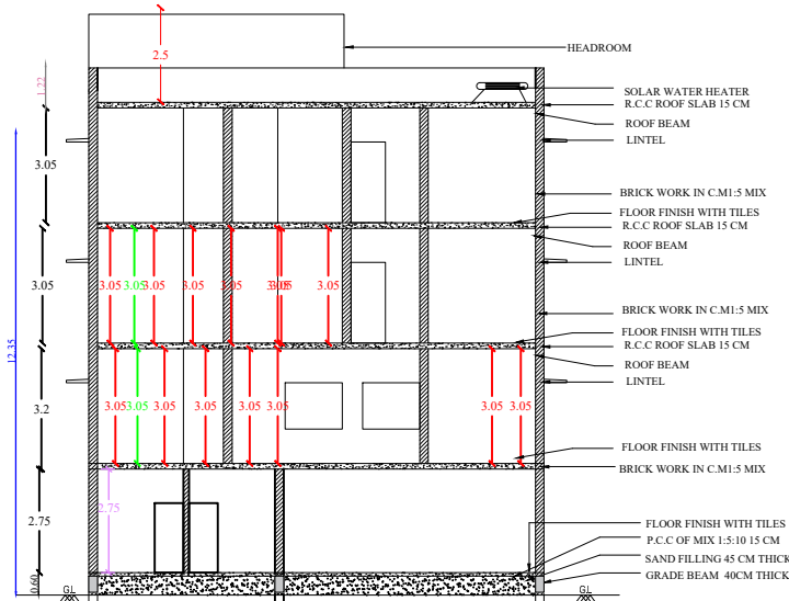
SECTION:A-B
