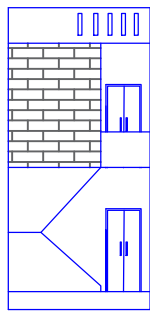
ELEVATION
