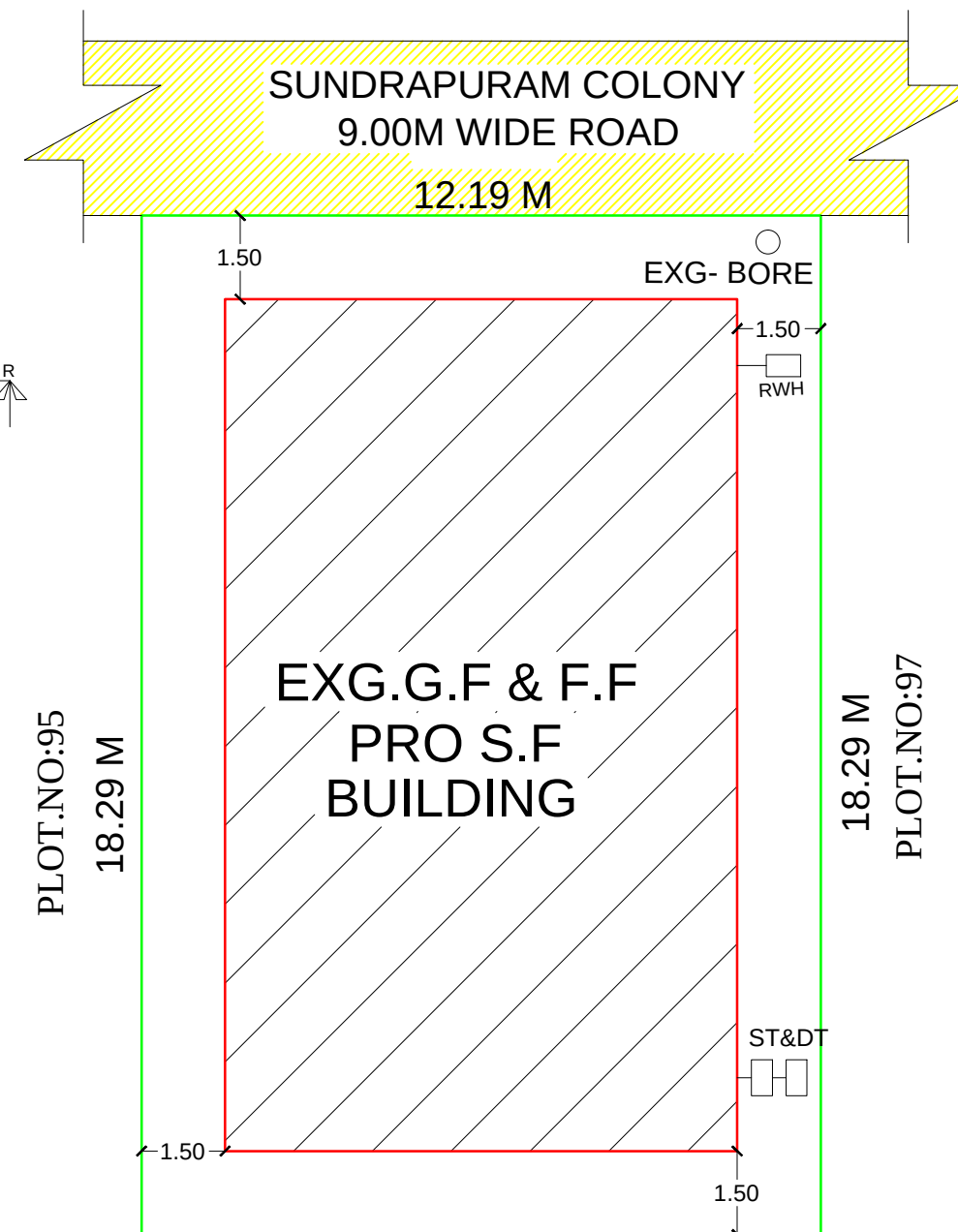
PLOT.NO:113 12.19 M SITE PLAN SCALE 1:100
