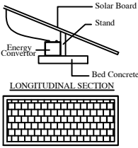
LONGITUDINAL SECTION
