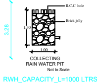
RWH_CAPACITY_L=1000 LTRS
