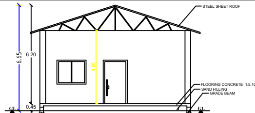
SECTION-AA R.S.NO:49/3A3A1 12.80
