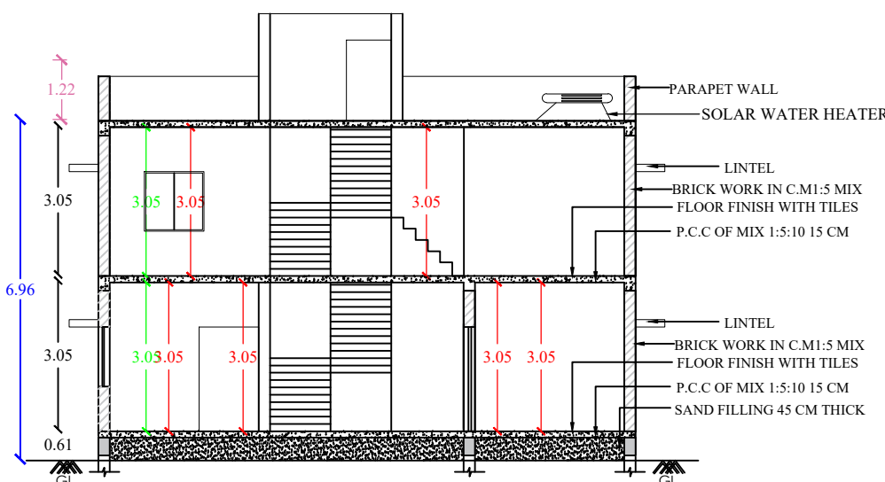
SECTION A-A
