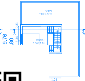
DOOR PLAN
