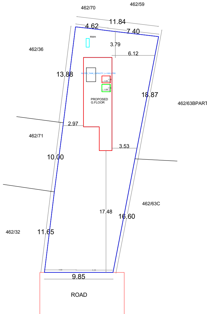
SITE PLAN 1:200
