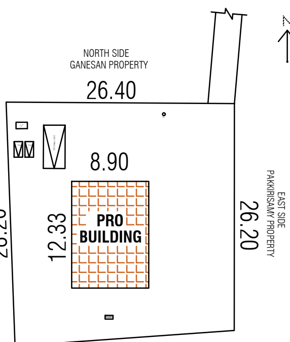
SITE PLAN SCALE- 1:400
