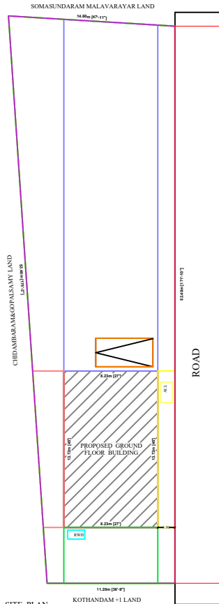
SITE PLAN SCALE: 1:100
