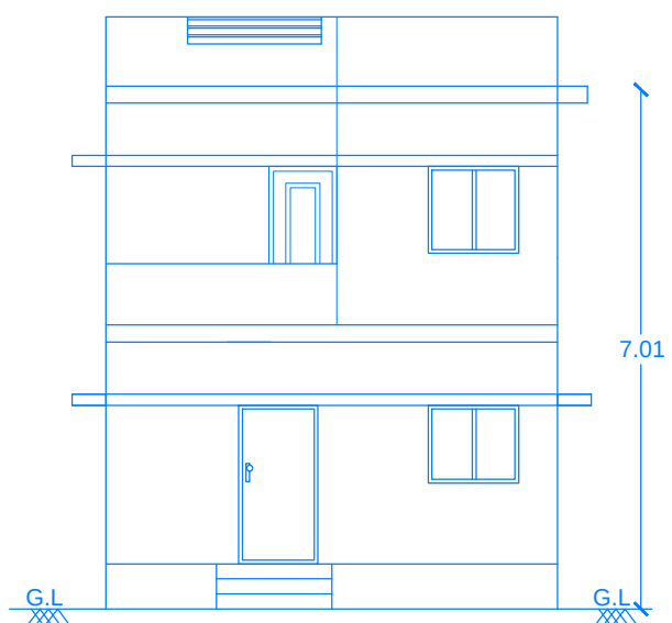
ELEVATION
