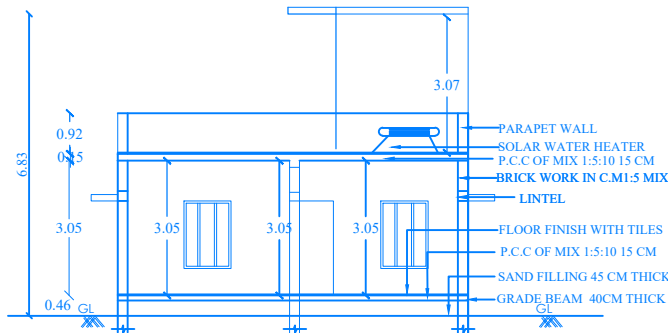
SECTION A-A1
