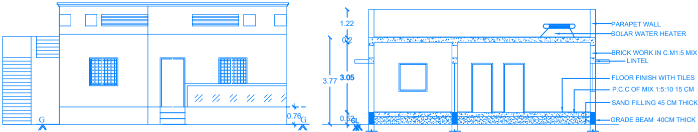
ELEVATION
