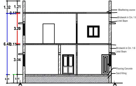
SECTION 'AB'
