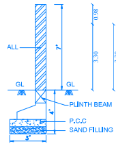
UND WALL DETAIL
