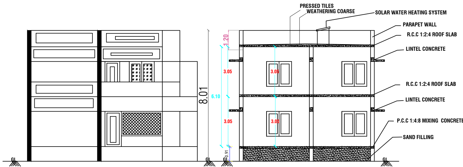
ELEVATION
