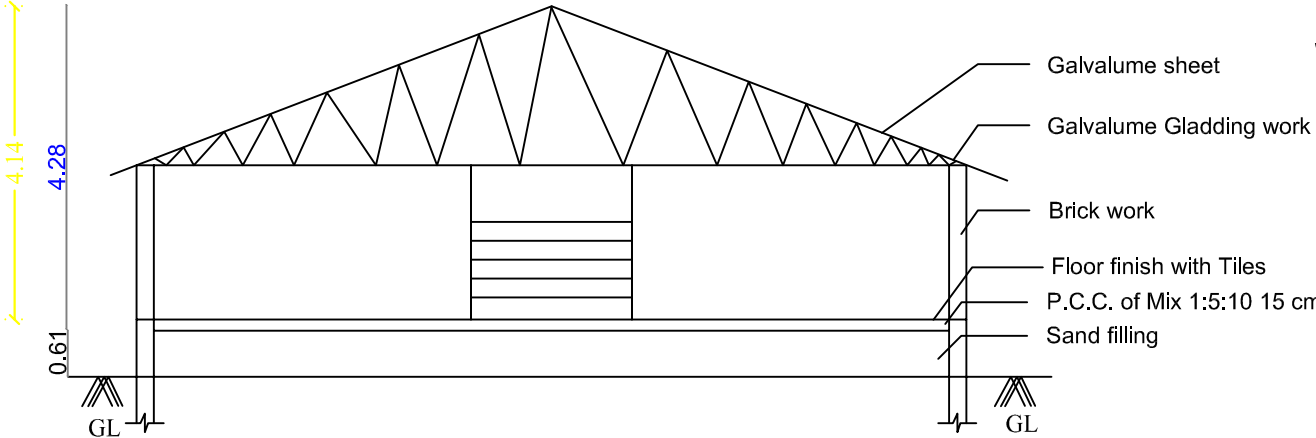
SECTION A-B
