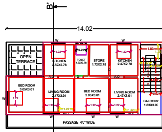
DOOR PLAN.
