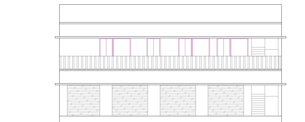
ELEVATION
