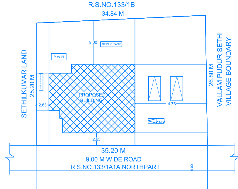
SITE PLAN SCALE 1:400
