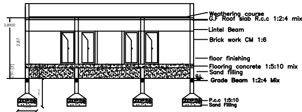
SECTION A-B
