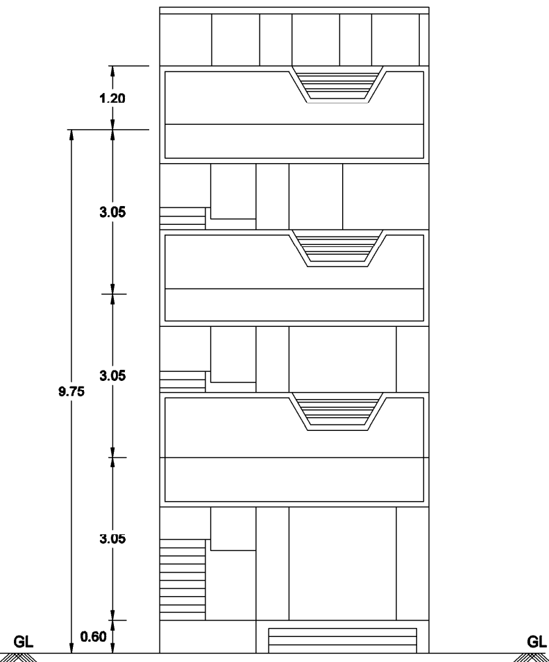
ELEVATION - A
