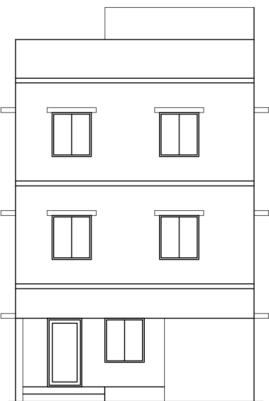
ELEVATION
