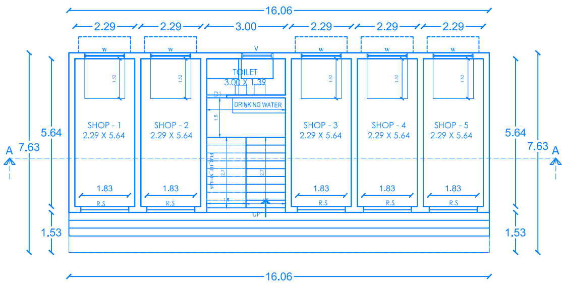
DOOR PLAN
