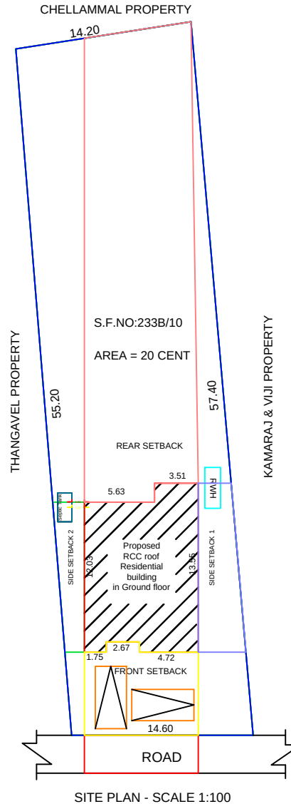
SITE PLAN - SCALE 1:100
