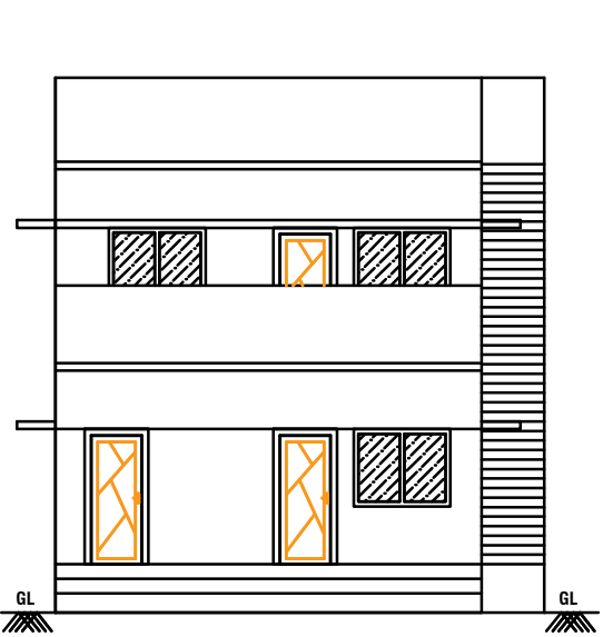
ELEVATION
