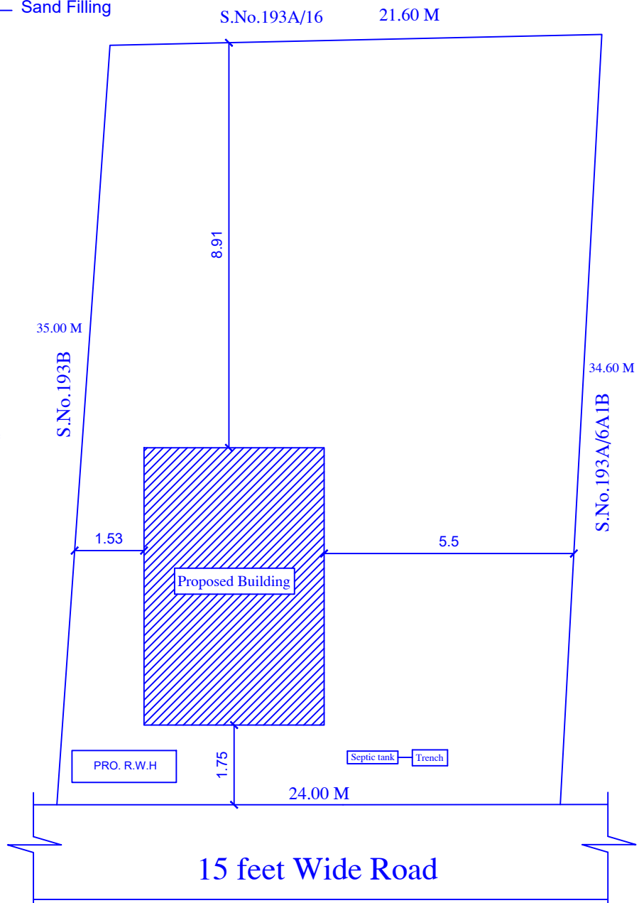
SITE PLAN 1:200
