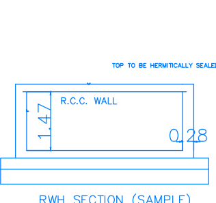
R.W.H. SECTION (SAMPLE)
