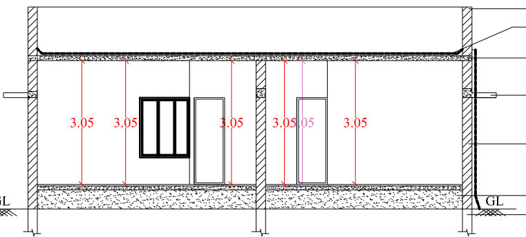
SECTION -XX
